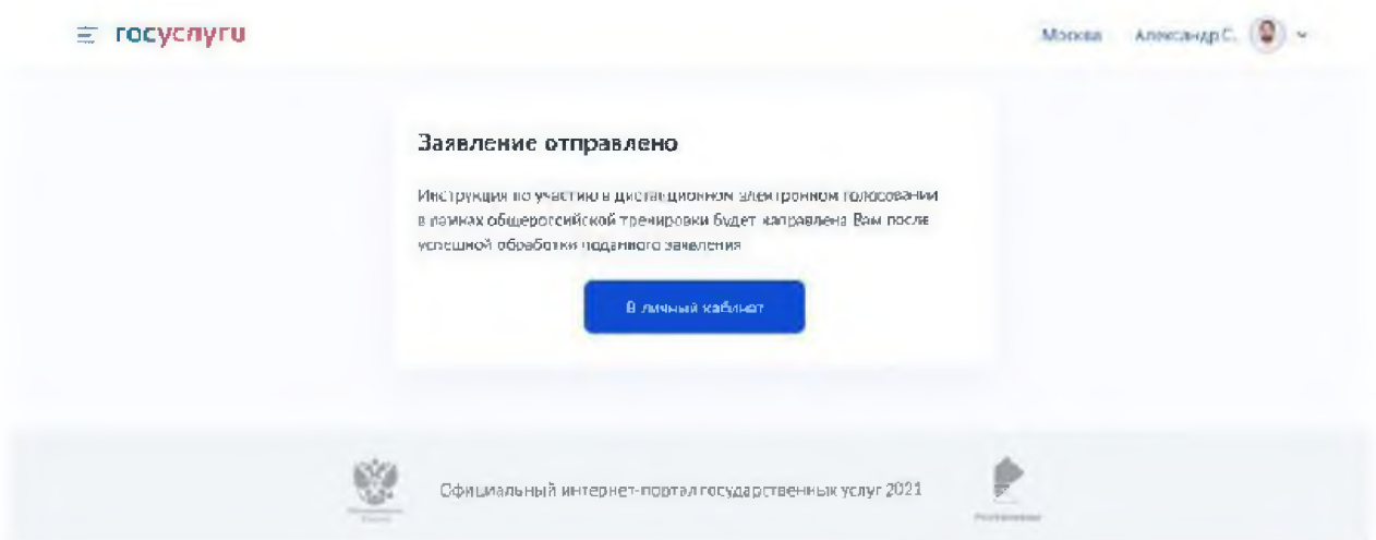
Рисунок 22 – заявление отправлено
